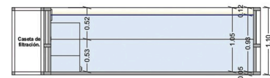
SECCIÓN B-B'.
