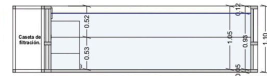
SECCIÓN B-B'.
