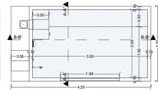
PLANO DE PLANTA Y ACCESORIOS.
